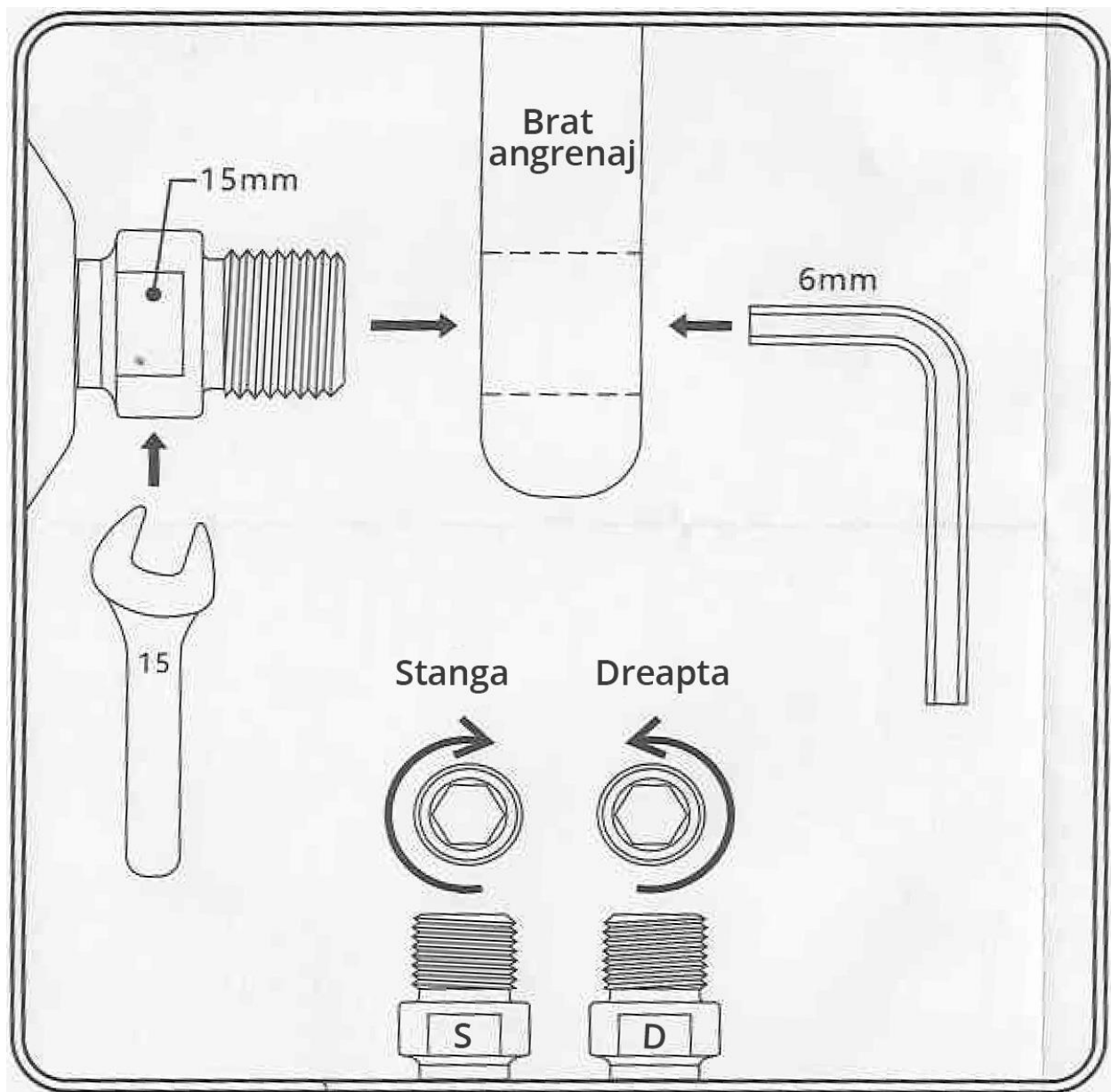
Montarea pedalelor
